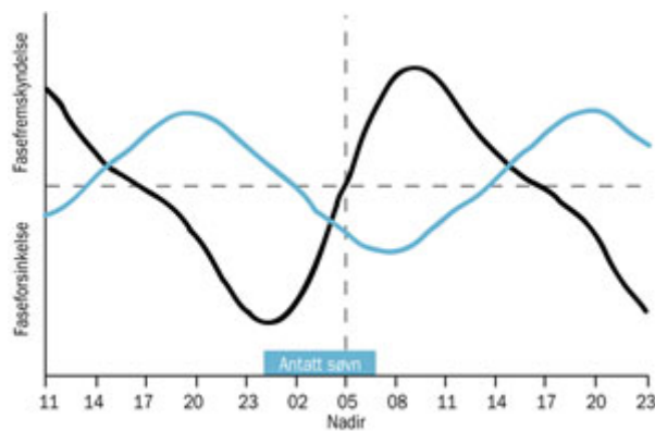
Figur 1. Fase-respons-kurve for lys (sort) og melatonin (blått) basert på studier av Khalsa et al. (2003) og Lewy et al. (1998). Forskjellen i styrken på effekten av lysterapi og melatonin vil ikke nødvendigvis være slik som det her er fremstilt, men vil være avhengig av lysintensitet, eksponeringstid og styrken på dosen av melatonin.
